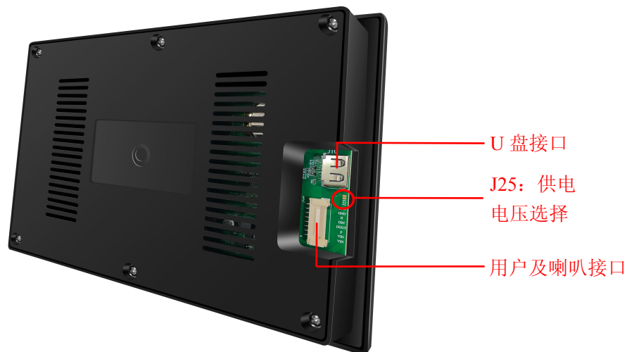
图 1 产品外观及硬件配置图
